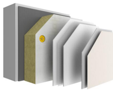
Nouveau système ITE StoTherm Mineral AimS® avec isolant en laine de roche
