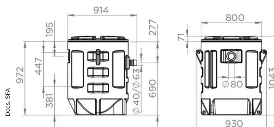
Sanifos 390 GR : prix publics indicatifs de 2 094 à 4 016 € selon modèle.
