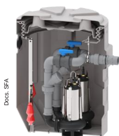
Sanifos 390 SLD, pour les eaux grises, eaux-vannes et eaux de pluie. Prix publics indicatifs de 1 928 à 4 292 € HT selon modèle.
