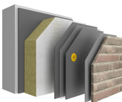
Système StoTherm Brick avec laine de roche
