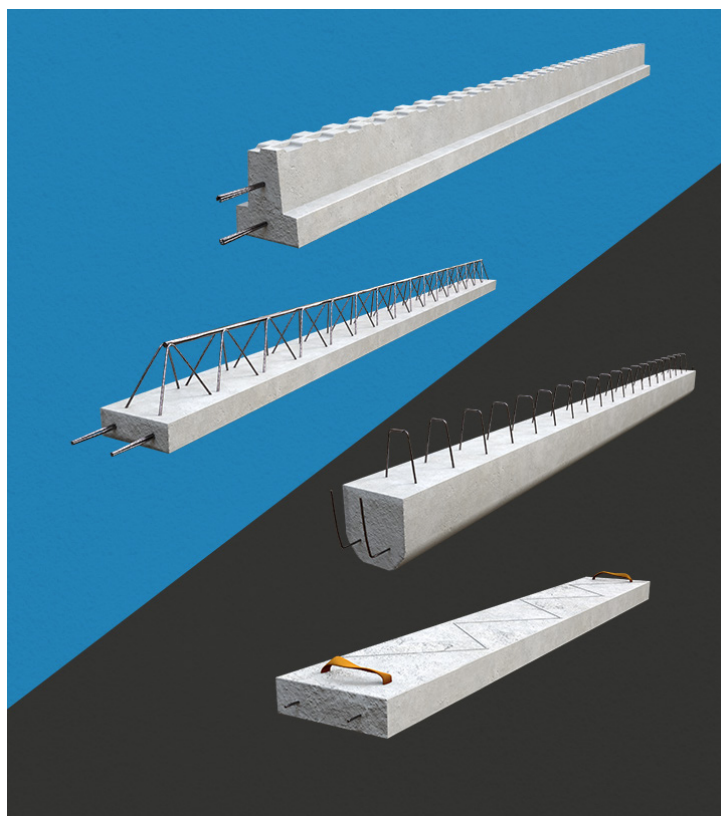
Gamme de poutrelles, poutres et prélinteaux EDILTECO®
