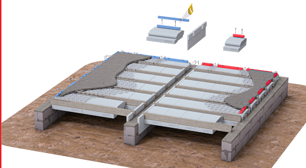
Système Global VS d'EDILTECO®
