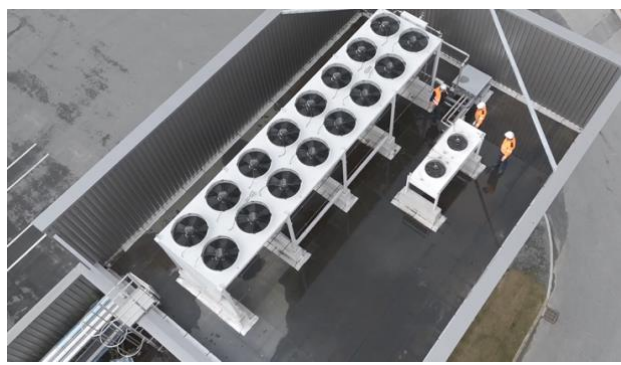
Un technicien Axima Réfrigération travaille sur les compresseurs du système
