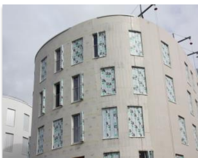
Le calepinage des plaques à enduire StoVentec, étudié en fonction de l'emplacement des 600 fenêtres, intègre 31 rayons de courbure différents. Crédit photo : Manuel Panaget
