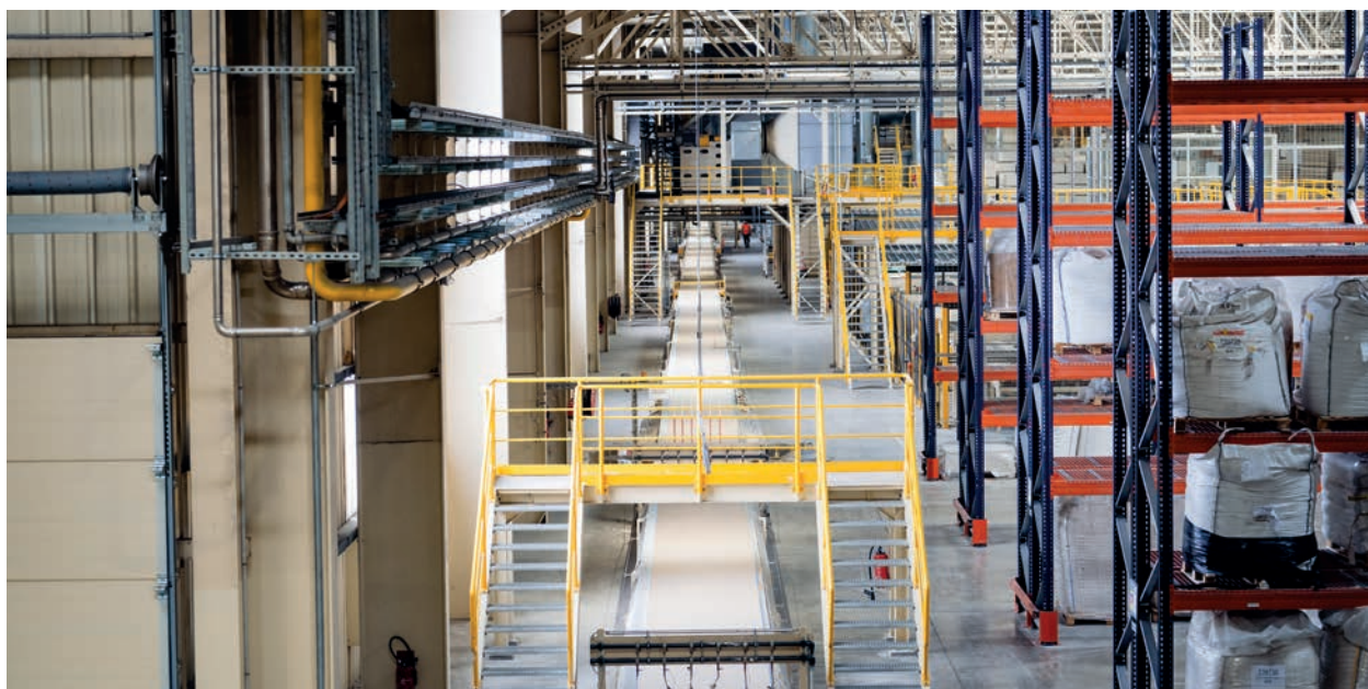
La nouvelle ligne de production de plaques de plâtre Knauf à Fos-sur-Mer, d'une capacité annuelle de 30 millions de m 2 .
