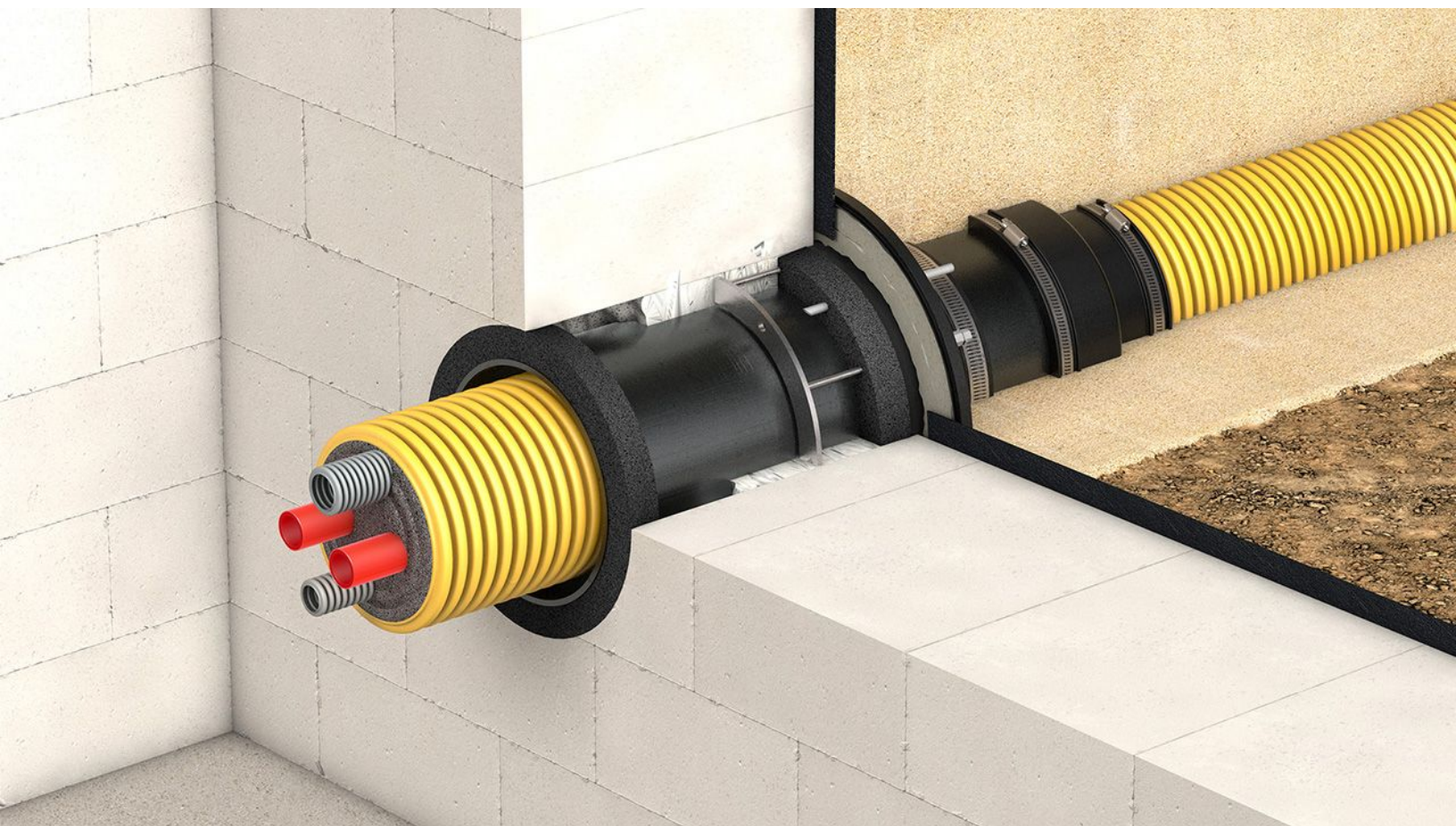
Le Quadro-Sicura® Quick/H/MAC en situation de montage ©DOYMA GmbH & Co
