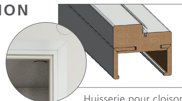
Huisserie pour cloison finie de 72 à 110 mm
