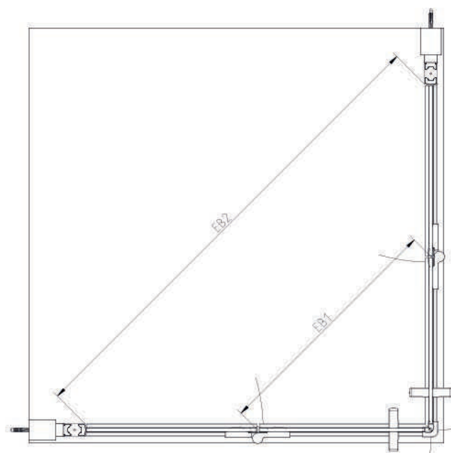
MI2CR + MI2CL = MONTAGE EN ANGLE LARGEURS D'ACCÈS
