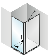
MIPIV + MIFXP p 269
