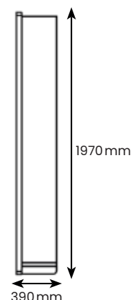
EITWA élément mobile
