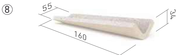
Inner transition corner Cantonera transición interior MDCA CI000 5.5x16
