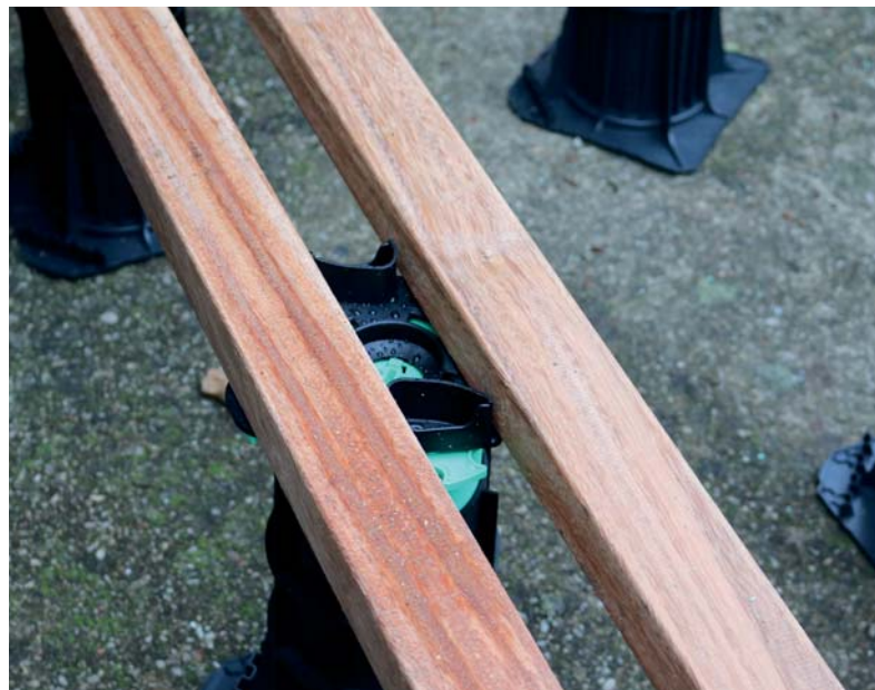
Double lambourdage possible avec une seule rangée de plots.
