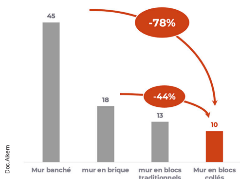
Poids carbone par m 2 de mur en eq. kg de CO 2
